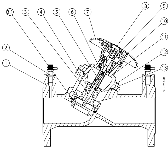
MSV-F2 DN 65
